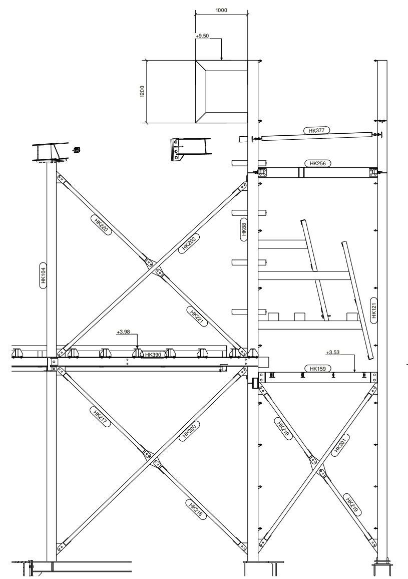
I - I
