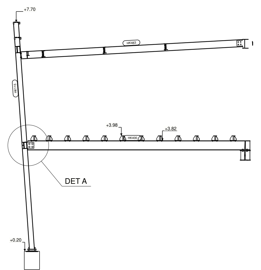
A - A
