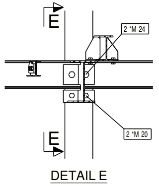
E - E
