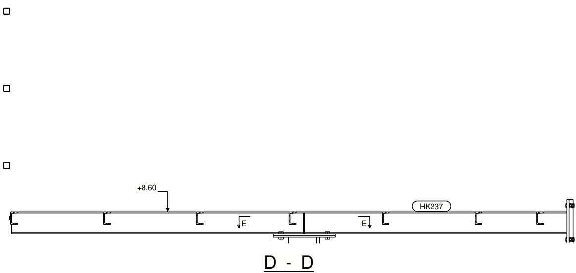
D - D
