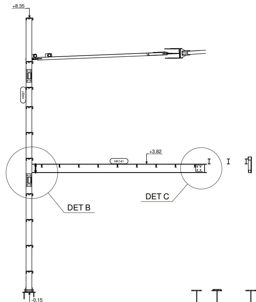
B - B
