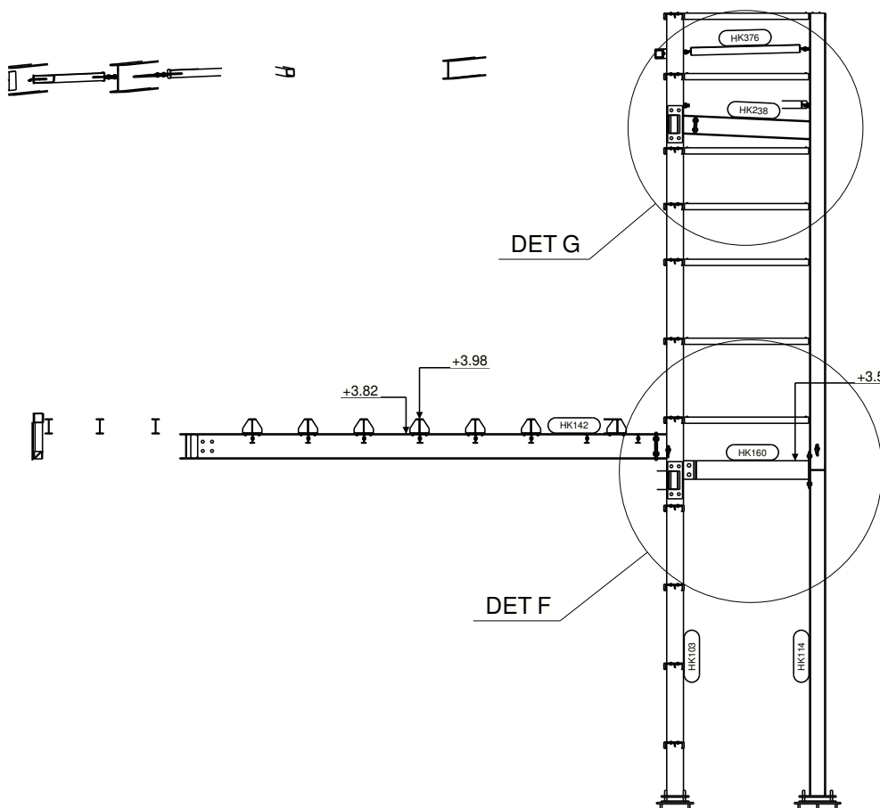
D - D
