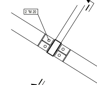
P - P
