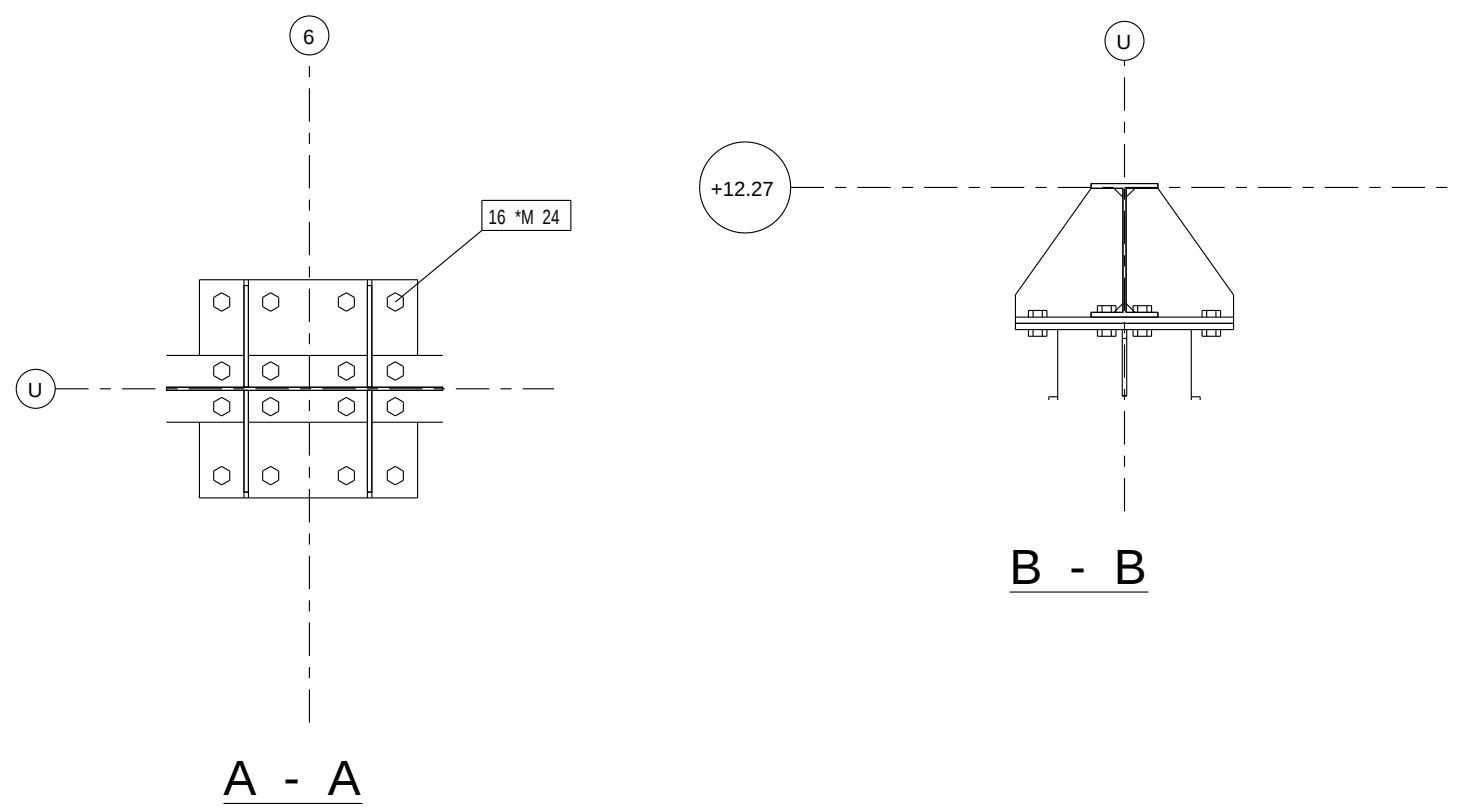
A - A
